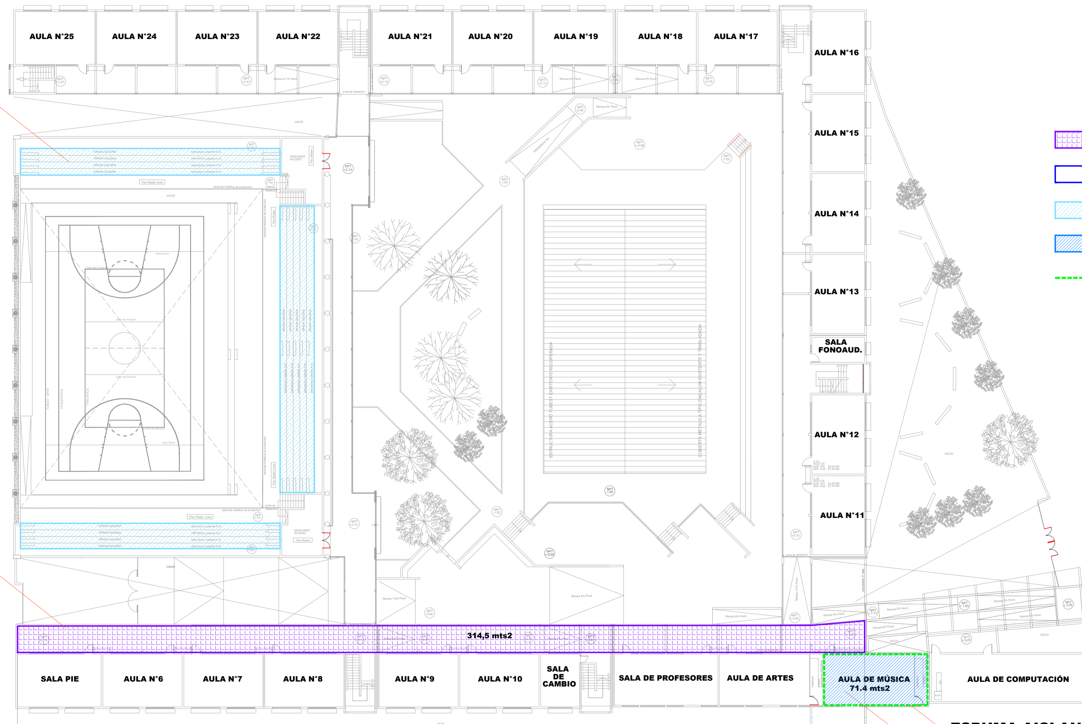
PLANTA DE ARQUITECTURA SEGUNDO NIVEL
