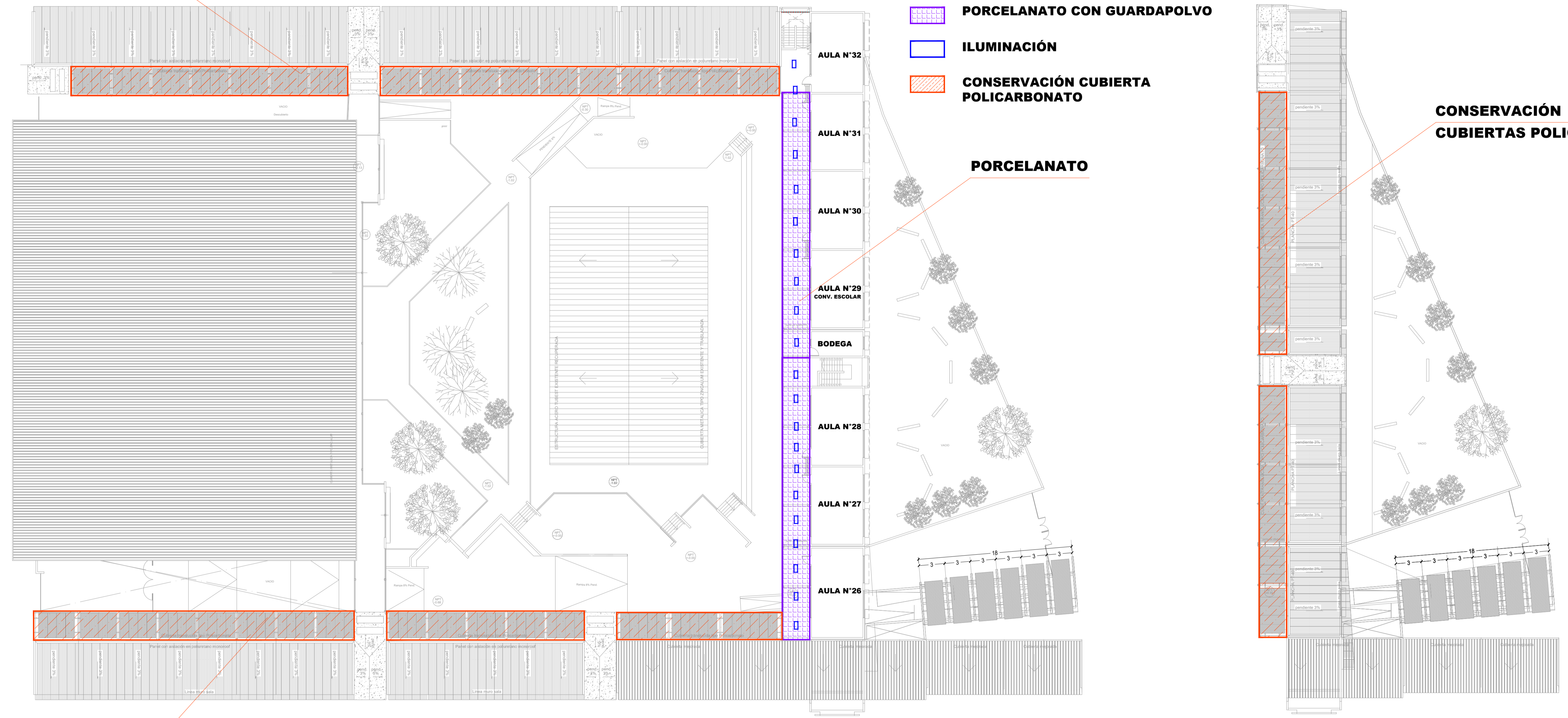
PLANTA DE ARQUITECTURA TERCER NIVEL
