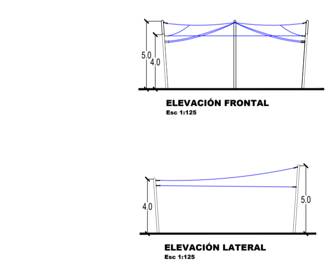
ELEVACIONES DE CUBIERTA HDPE
